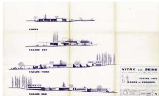
Coupe et façade d'un centre aéré de Vitry (1971) Fonds Contrôle de la légalité du Val-de-Marne 1184W 102
