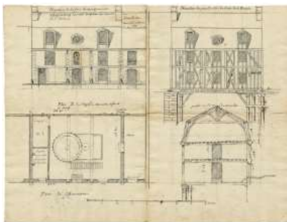
Plan du Moulin Saint-Antoine situé sur le pont de Charenton (XVIIe siècle) Fonds Malon de Bercy 46J 71
